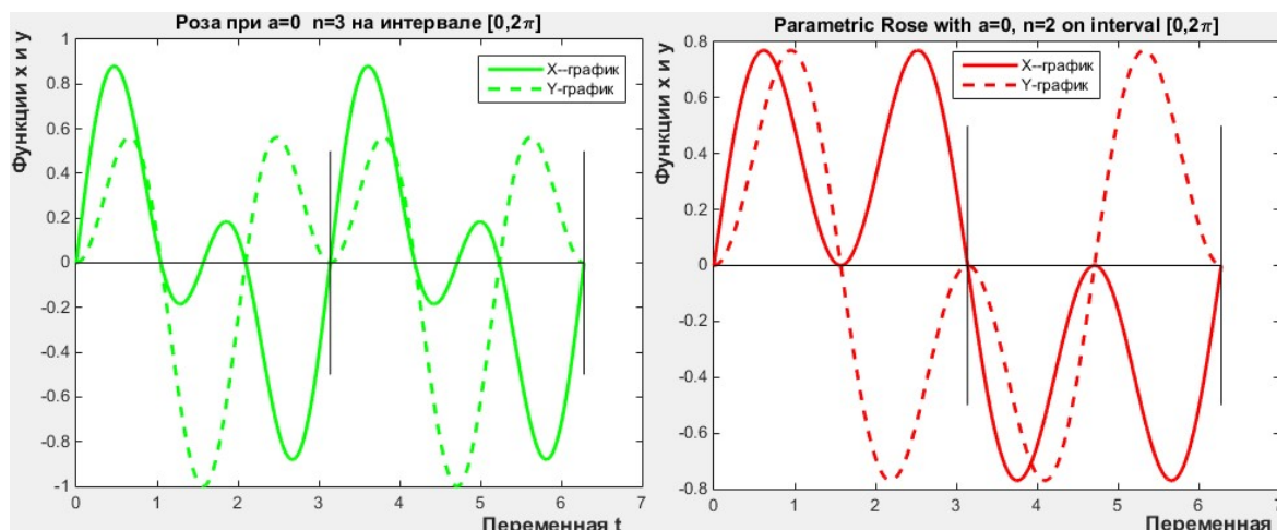
Рис. 3. Поведение ветвей розы (1) при нечетном (слева) и четном n (справа), полученное программой Learn1RoseCoeff
