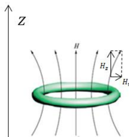
Рис.3 Компоненты силовых линий
