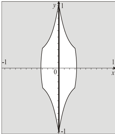
Рис. 1. Області коректності (біла) та некоректності (сіра) наближення рівномірно зарядженої нескінченної нитки при \varepsilon_E = 5\% , \delta_\alpha = 5^\circ
