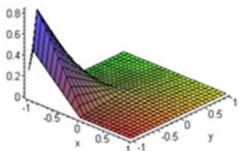
Рис. 4. Графік n_1(x, y)
