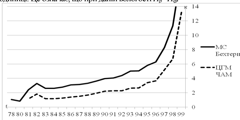
Рис.1 Графік залежності перевідного коефіцієнта К від відносної вологості повітря f для ЦГМ ЧАМ(м. Одеса) та МС Бехтери (Херсонська область)
