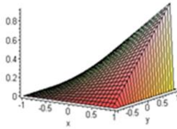
Рис. 8. Графік h_4(x, y)
