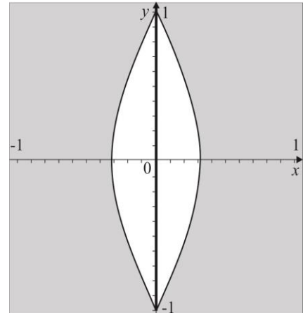
Рис. 3. Області коректності (біла) та некоректності (сіра) наближення нескінченно довгого прямого провідника зі струмом при \varepsilon_B = 5\% .
