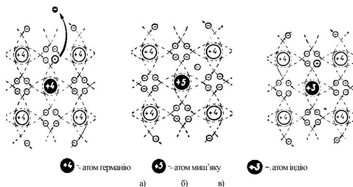
Рис. 2. Таблиця «Види провідності германію» : а) електронно-діркова (власна); б) електронна (домішкова); в) діркова (домішкова).
