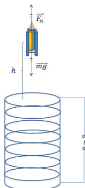
Рис.8. Космический корабль в положении равновесия над катушкой
