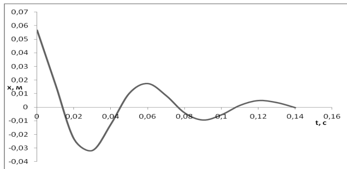
Рис.3. График зависимости координаты от времени
