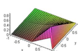
Рис. 6. Графік n_3(x, y)
