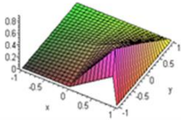
Рис. 7. Графік h_3(x, y)
