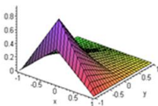
Рис. 5. Графік n_2(x, y)
