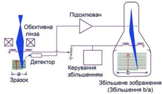
Рис. 2. Принцип роботи скануючого електронного мікроскопа
