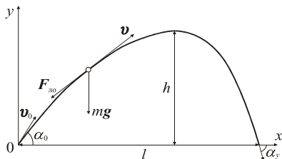
Рис. 1. Рух тіла, кинутого під кутом до горизонту з урахуванням сили лобового опору повітря
