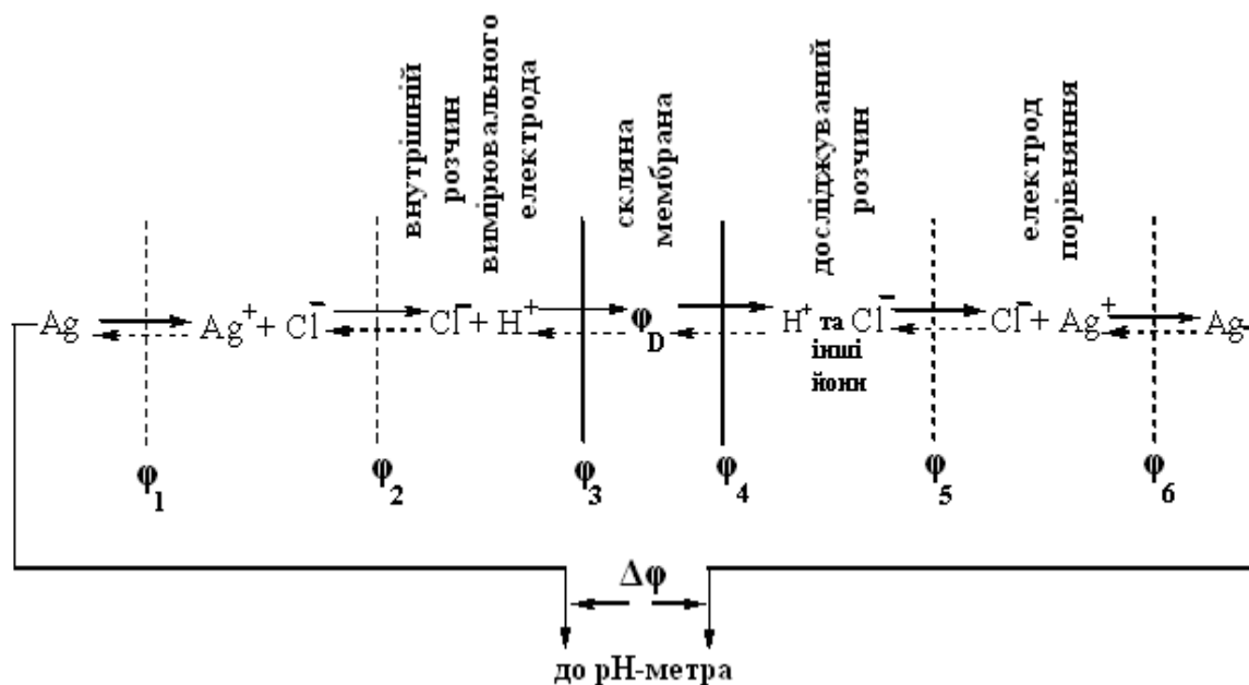
Рис. 7. Електрохімічний ланцюг. \phi_4 описується законом Нернста.
