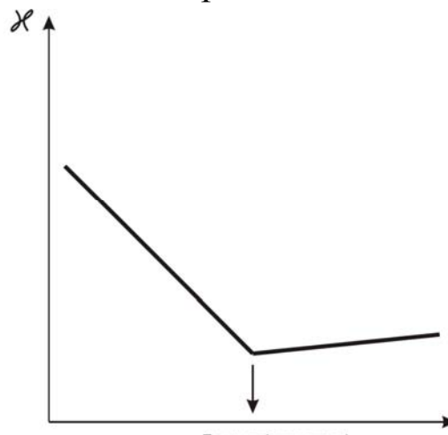
Крива кондуктометричного титрування сильної кислоти слабкою основою
