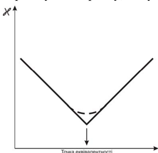
Крива кондуктометричного титрування сильної кислоти сильною основою
