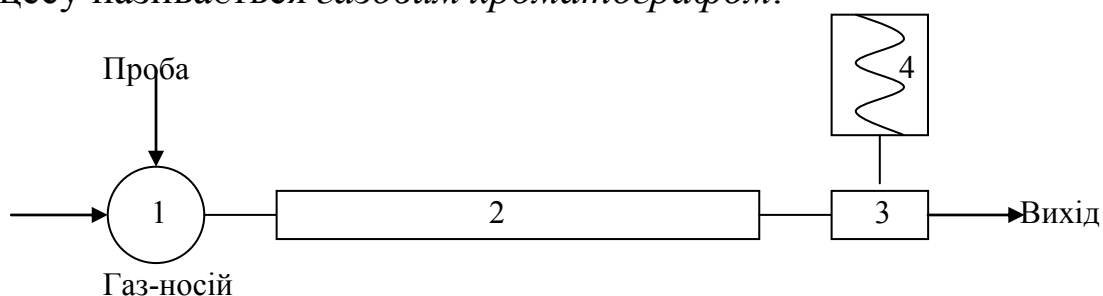
Рис. 11. Принципова схема газового хроматографа.
