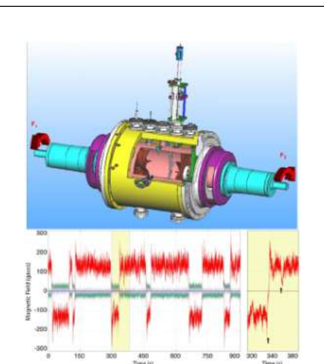
Прилад, який дозволив реконструювати інверсії магнітного поля Землі. В ході експерименту, розплав металу за допомогою спеціальних насосів обертався навколо металевого стержня. При цьому генерувалися електричні струми і формувалося магнітне поле, перпендикулярне потоку заряджених частинок. Прилад реєстрував спонтанні флуктуації магнітного поля, які аперіодично завершувалися змінною магнітних полюсів в даній моделі.
