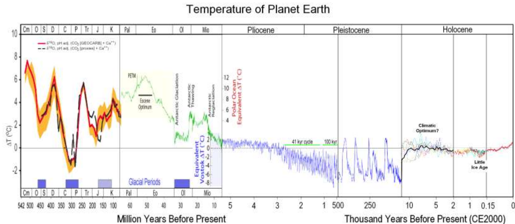
Рис. Динаміка температур навколишнього середовища в Фанерозої. Де: осі ОХ – геологічний час, млн. р.т. (Кембрій –Пліоцен); тис. років тому (Плейстоцен-Голоцен); по осі ОУ – температура навколишнього середовища; Cm – Кембрій, О – Ордовик (масове вимирання видів наприкінці Ордовика \approx 440 млн. років тому; різке похолодання клімату); S – Силур; D – Девон (масове вимирання видів в Девоні \approx 365 млн. років тому; різке потепління клімату); C – Карбон; P – Пермь (масове вимирання видів в Пермському періоді \approx 250 млн. років тому; різке похолодання клімату); Tr – Тріас (масове вимирання видів в Тріасі \approx 215 млн. років тому; різке потепління клімату); J – Юра; K – Крейда (масове вимирання видів в Крейдяному періоді \approx 65 млн. років тому; падіння великого астероїда).
