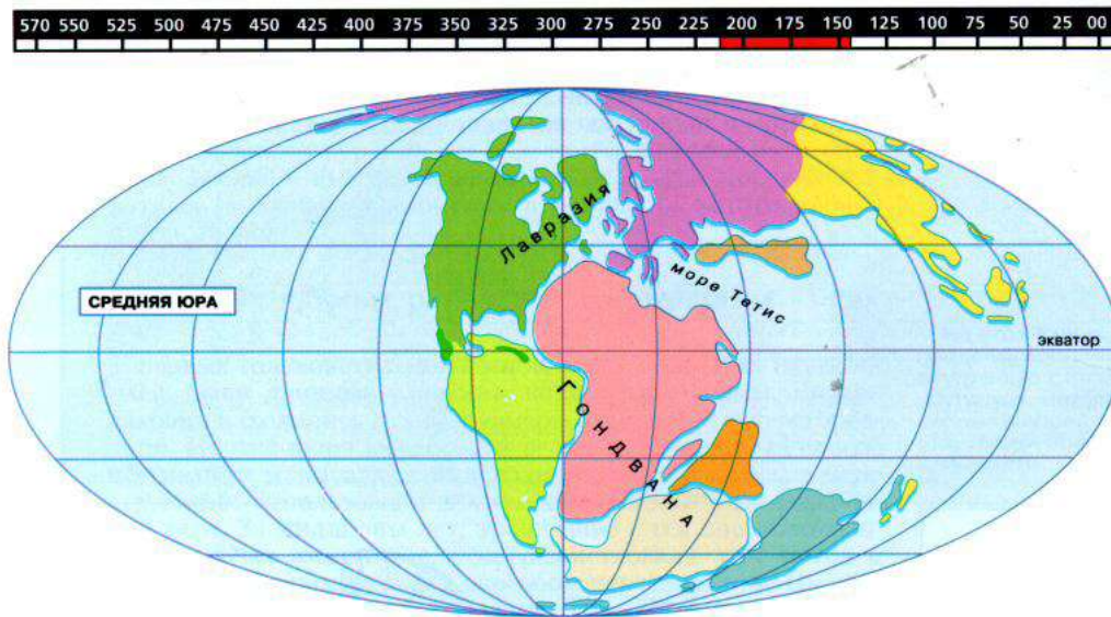
Рис. 1 А. Розташування континентів в середині Юрського періода.
