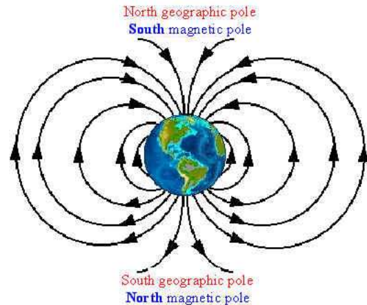
Магнітне поле Землі має і постійну, і змінну компоненти.
