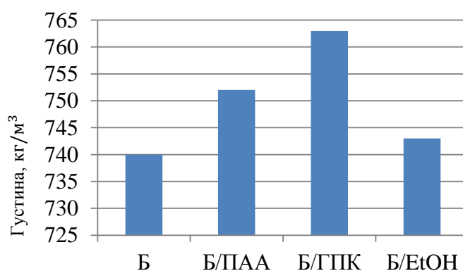
Рис.7. Залежність густини бензину марки А-92 від природи активатора згорання (5% мас.): Б-бензин А-92, Б/ПАА-суміш бензину та параацетальдегіду, Б/ГПК-суміш бензину та гідропероксиду кумолу, Б/EtOH-суміш бензину та етилового спирту).
