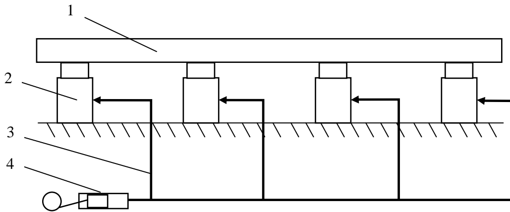
Рис.-1. Схема гідравлічної системи відкривання трюмів де 1 – кришка трюму; 2 – гідравлічний домкрат; 3 – гідравлічний трубопровід; 4 – гідравлічний плунжерний насос
