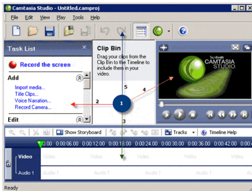
Рис. 1. Вікно програми Camtasia Studio. 1 – Робочий стіл. 2 – Панель управління. 3 – Шкала часу. 4 – Програвач. 5 – Панель інструментів.
